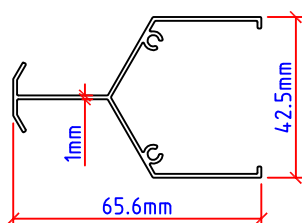
LK5827 Scale 1:2
