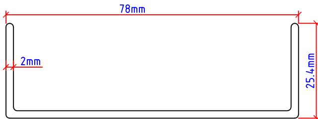
3986 Scale 1:1
