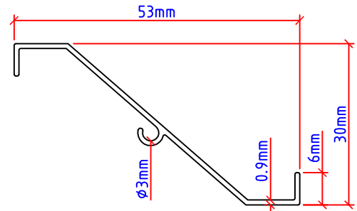
FB222 Scale 1:1
