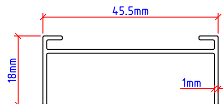
LK5828 Scale 1:1
