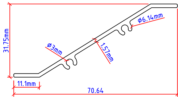
AA563 Scale 1:1
