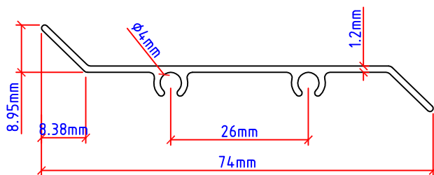
SJ163 Scale 1:1
